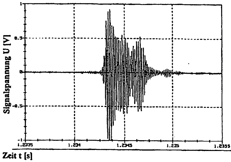
Kontinuierliche Schallemission infolge Gelenkreibung
